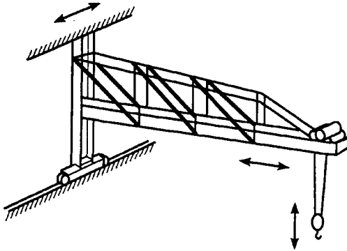
FIG. 5 WALL CRANE
